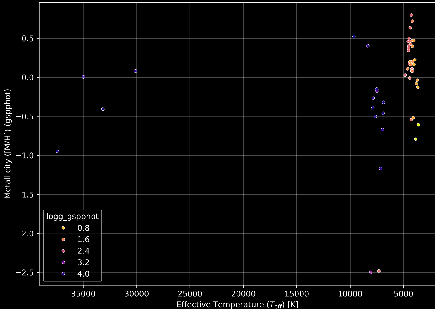
APOGEE DR17 Field: [279-33-O] Stellar Population Parameters (n= 56)
